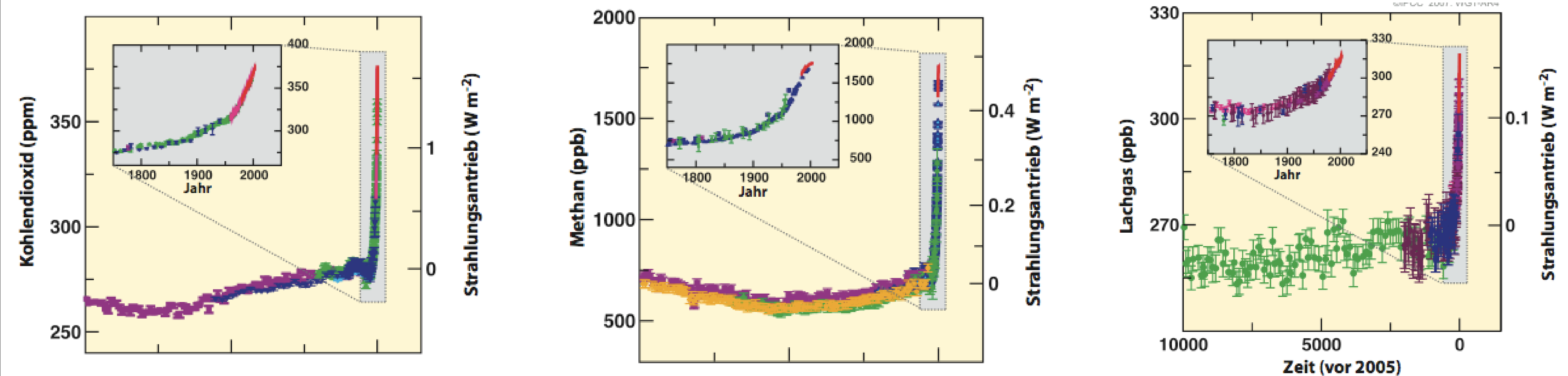
ABBILDUNG SPM.1. Atmosphärische Konzentrationen von Kohlendioxid, Methan und Lachgas in den letzten 10'000 Jahren (große Grafiken) und seit 1750 (eingefügte Grafiken). Dargestellt sind Messungen aus Eisbohrkernen (Symbole mit verschiedenen Farben für unterschiedliche Studien) und atmosphärischen Proben (rote Linien). Die entsprechenden Strahlungsantriebe sind auf der rechten Achse der großen Grafiken angegeben. (Abbildung 6.4)
